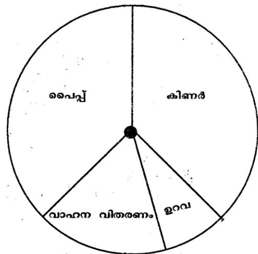
വരൾച്ച മാസത്തിൽ കുടിവെള്ള സ്രോതസ്സ്
